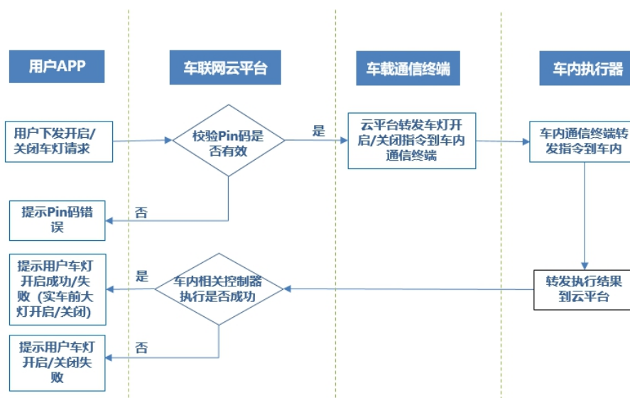
图 A.4 远程车灯控制业务流程
