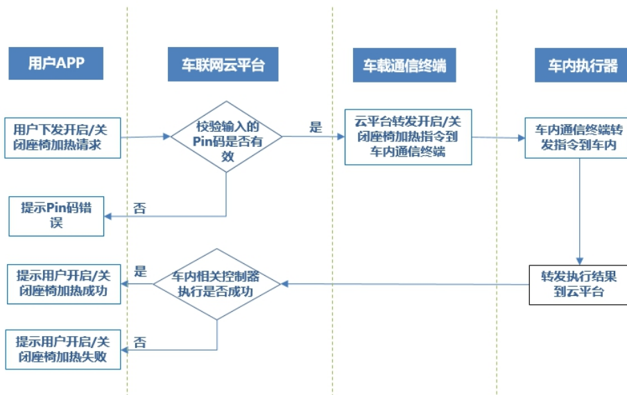
图 A.3 主驾/副驾/左后/右后座椅加热开启/关闭业务流程图
