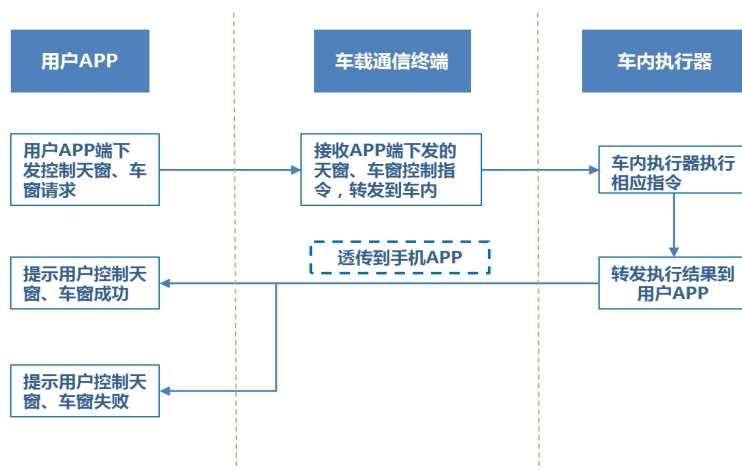
图 2.9 车窗、天窗控制业务流程图
